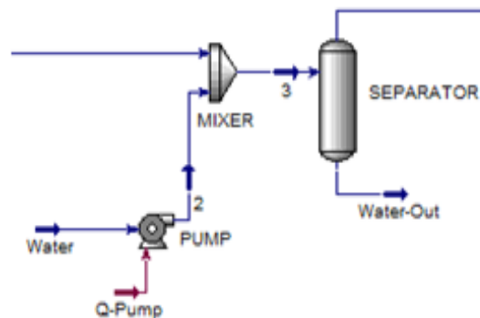
Figure4. Fogging Unit
